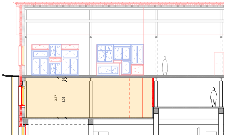
Schnitt AA
