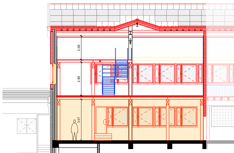
Schnitt AA
