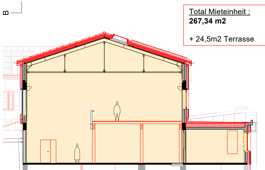
Schnitt BB
