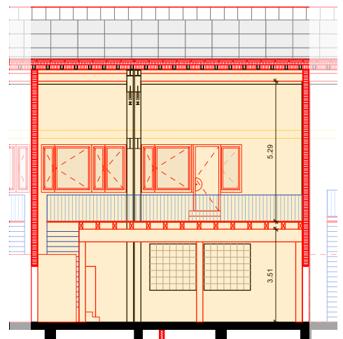
Schnitt AA
